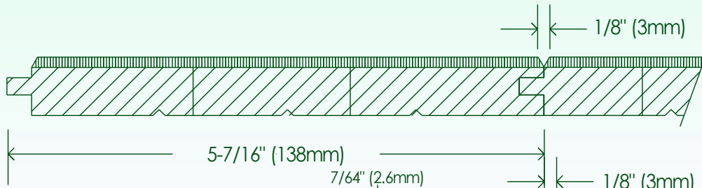
MICRO-V 122-041-000
